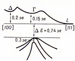
Рис. 3. Схема энергетических зон Ge; \Delta\mathcal{E} — ширина запрещенной зоны, L, Г и Δ — три минимума зависимости \mathcal{E}(p) в зоне проводимости вдоль осей [100] (L), Г и [111] (Δ).
